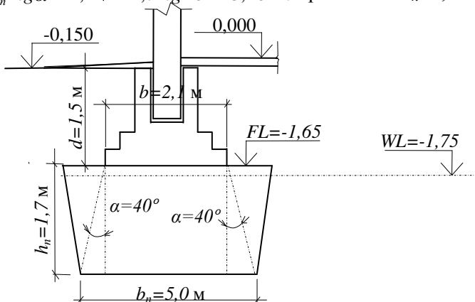
Рис. 6.1 До розрахунку піщаної подушки
